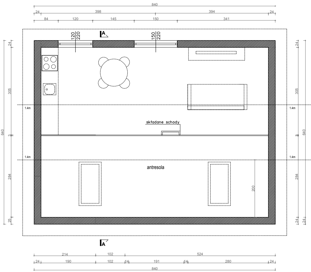
ENTRESOL PLAN
